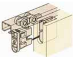
ソフトクローズ機構付上吊引戸用レールセット (2way仕様) RDT-001HR2W(35mm厚ドア用) ¥21,000/セット ※引戸は2セット必要となります。
